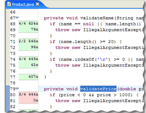
(d) Coverage View
