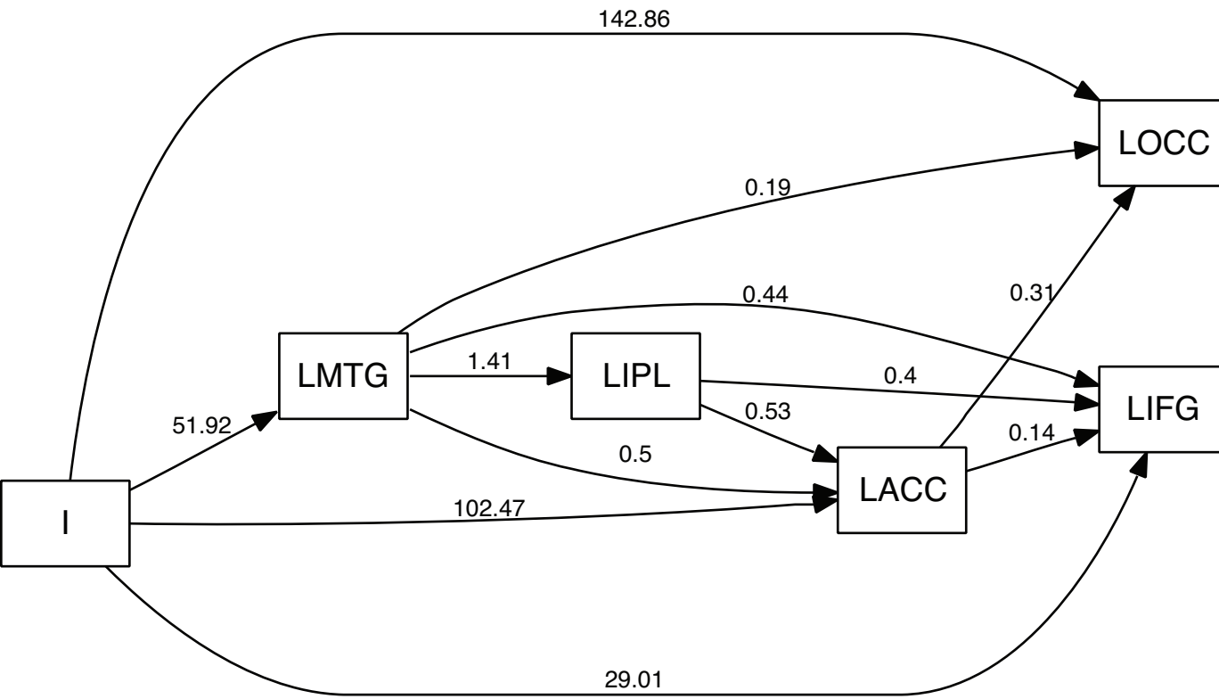
B: SEM (using modification indices)
