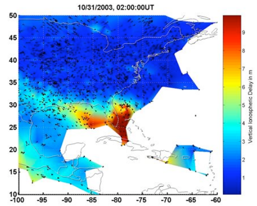
(d) 02:00 UT (21:00 EST).
