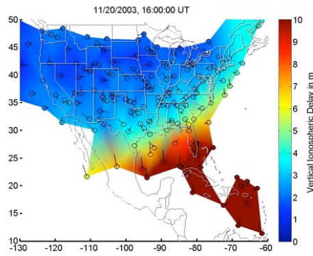
(i) 16:00 UT
