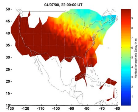
(l) 22:00 UT
