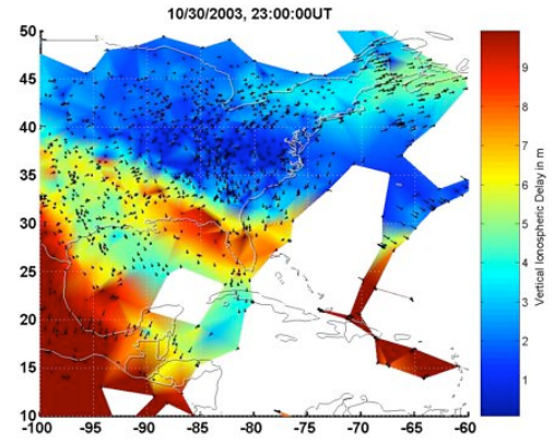
(b) 23:00 UT (18:00 EST).
