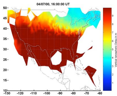
(i) 16:00 UT
