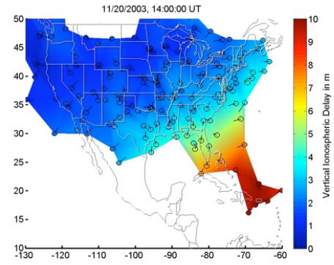
(h) 14:00 UT
