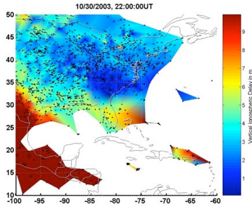
(a) 22:00 UT (17:00 EST).
