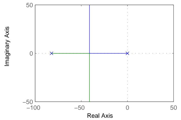
Root locus for G2 = 10
