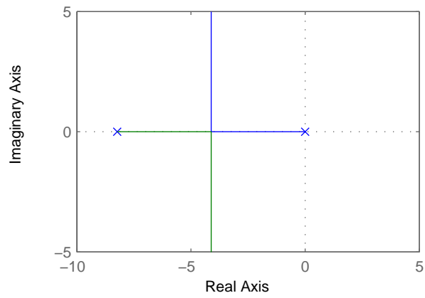
Root locus for G2 = 1
