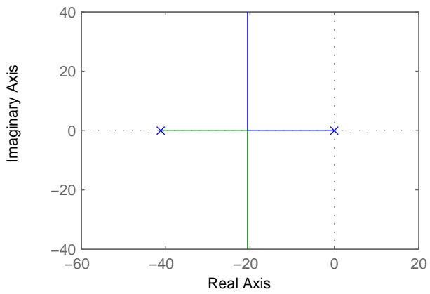
Root locus for G2 = 5
