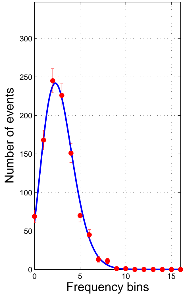
Poisson simulator
