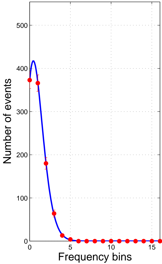
Poisson simulator
